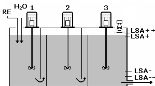
Рис. 12.1 Принципиальная схема работы
